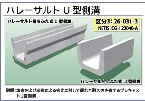
写真1：製品形状
